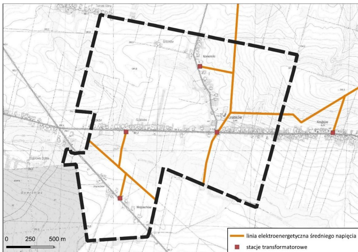
Rysunek 9. Przebieg linii elektroenergetycznych na terenie opracowania
